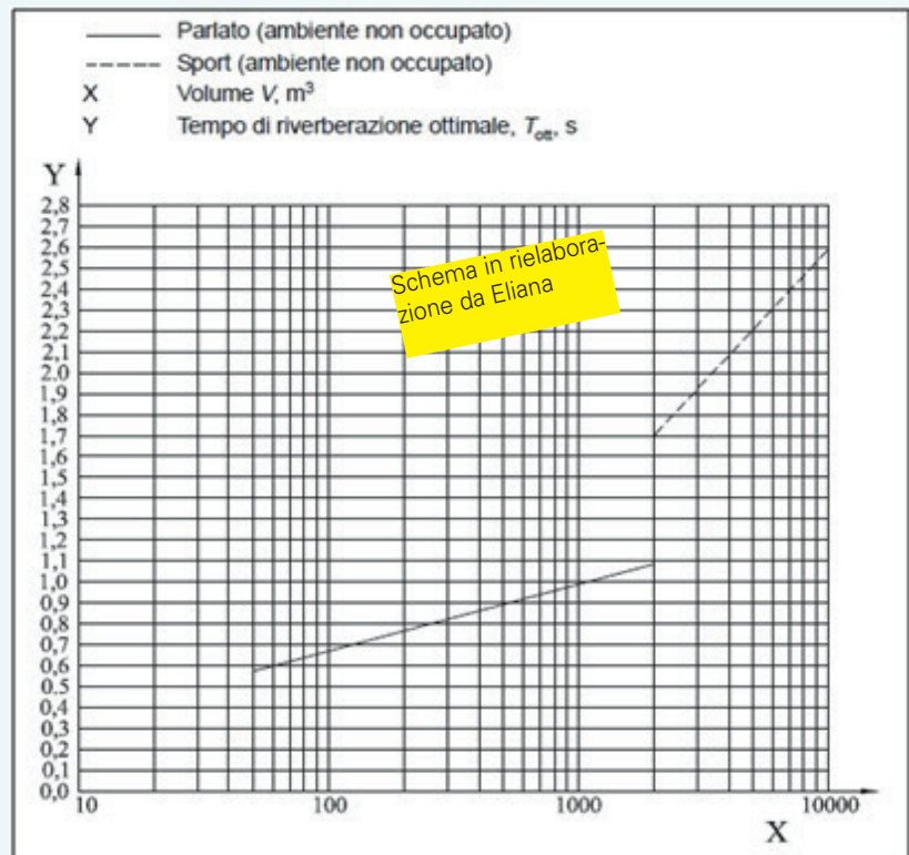
Fig. 1 Tempo di riverberazione ottimale in funzione del volume V
